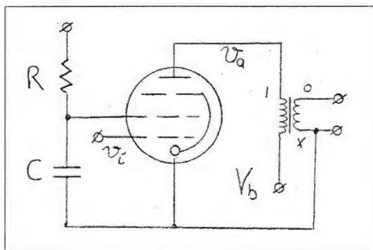
fig.29 Gedeeltelijk-kathode-gekoppelde schakelwijze.
